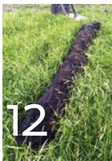
Subfossiele veeneiken
